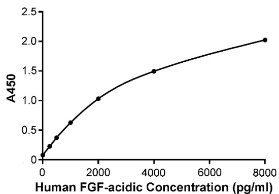
图3. Human FGF-acidic ELISA Kit的标准曲线。实测数据会因实验条件、检测仪器等的不同而存在差异，图中数据仅供参考。
